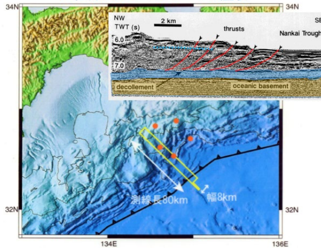
付図 9-土佐沖メタンハイドレートの産状
