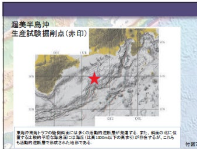
付図 7-渥美半島沖の生産試験掘削地点
