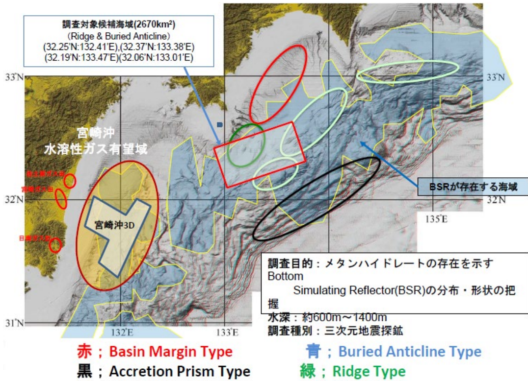
付図 13-高知沖付加帯におけるメタンハイドレート分布域の三次元地震探鉱探査
