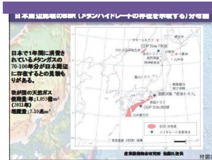
付図1-日本周辺海域のメタンハイドレート分布図
